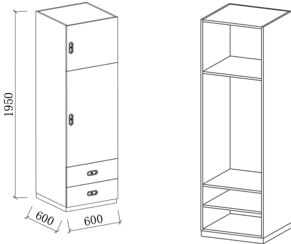
图 11 衣柜（两门衣柜）示意图
