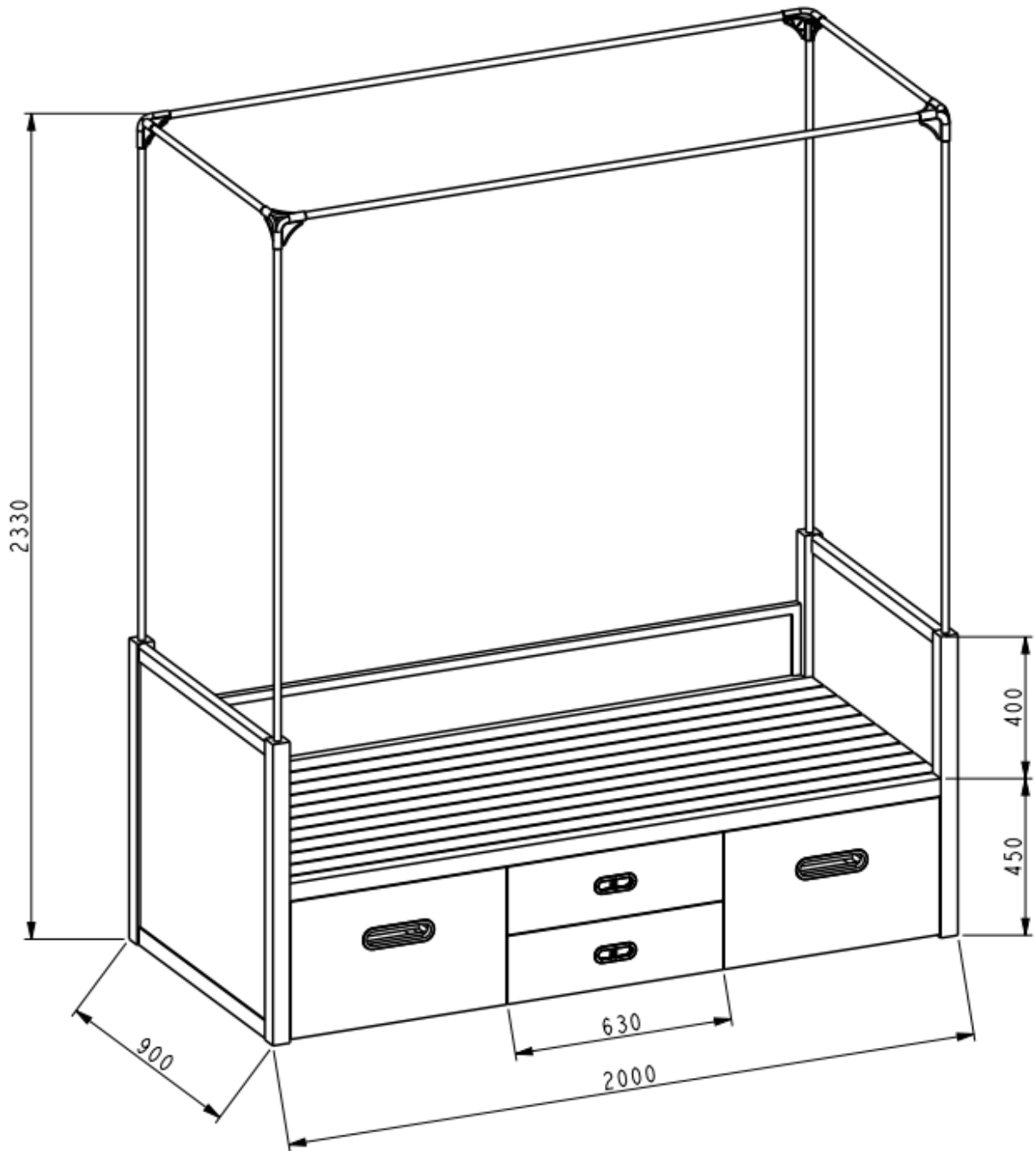
图 9 单人床示意图
